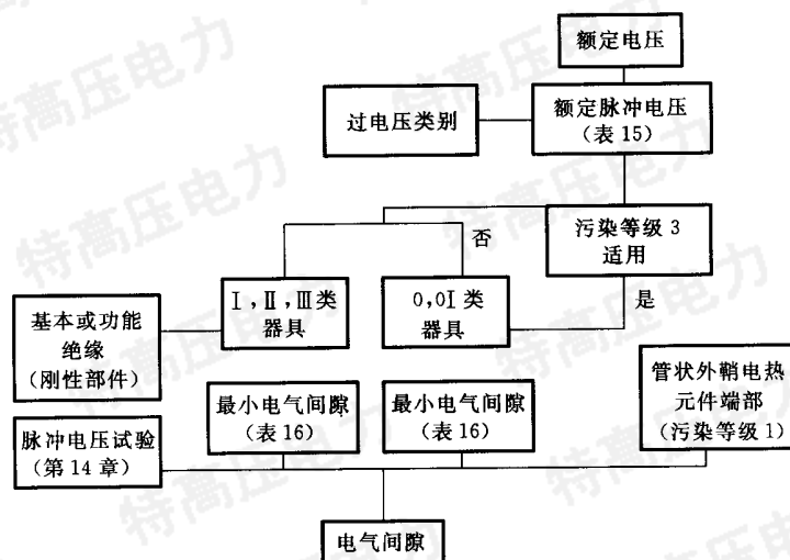
图 L.1 测定电气间隙的程序
