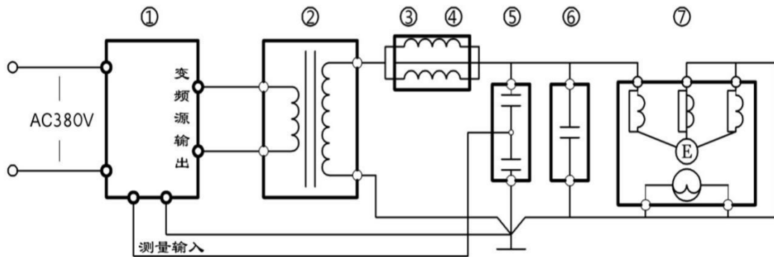
发电机耐压试验接线图
