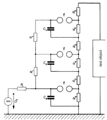
图 1 Marx 回路 (3 级) 示意图
