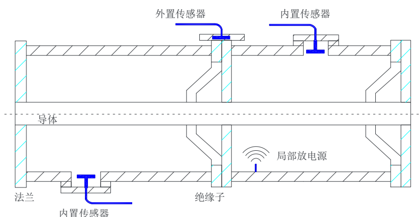
图 3-3 特高频测量原理图
