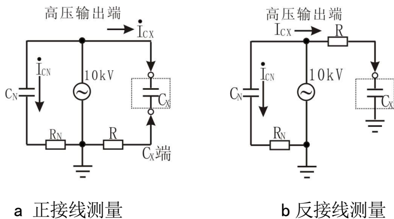
图 3 测量原理图
