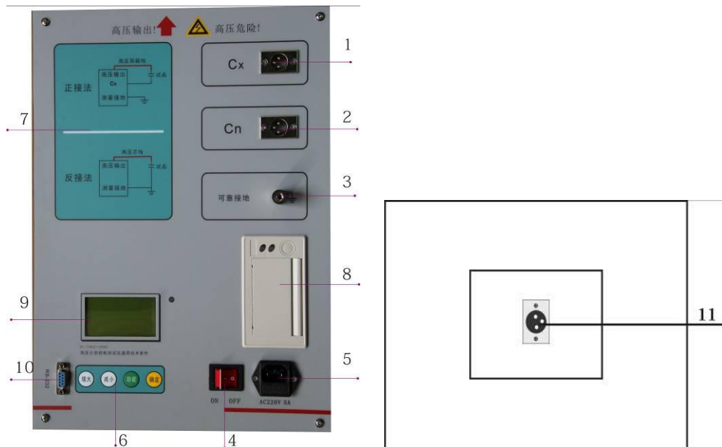
图 1 仪器面板和侧面
