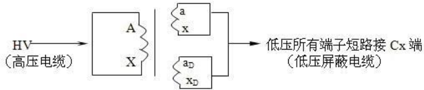
图 7 常规接线法
