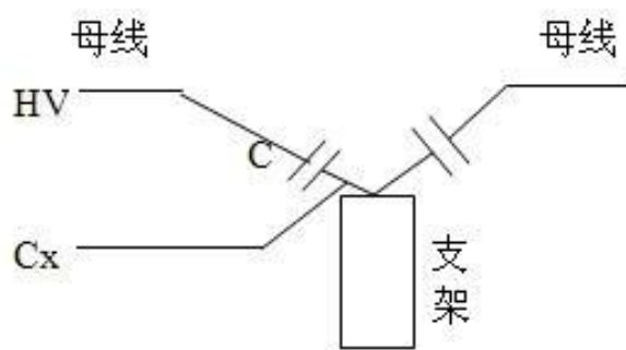
图 10 断路器断口电容试验接线
