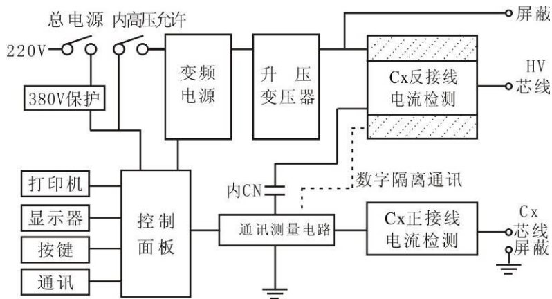
图 2 仪器结构图
