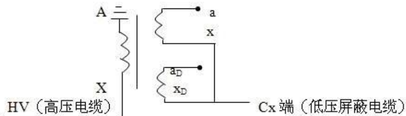
图 9 末端加压法接线
