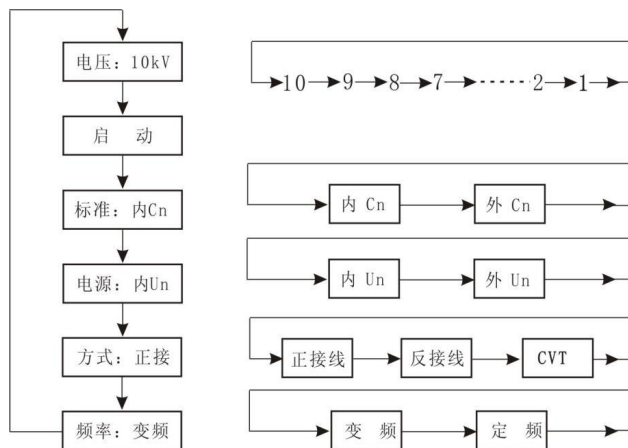
图 21 光标移动流程图 图 22 菜单内容选择
