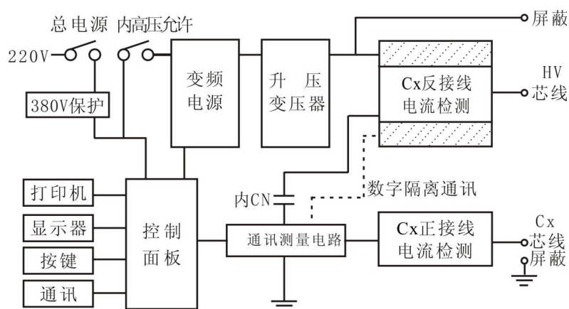
图 2 仪器结构图
