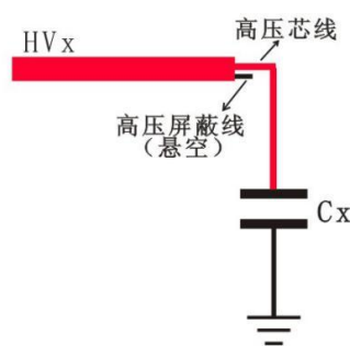
图 6 反接法
