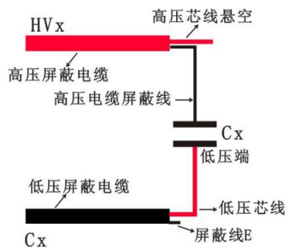
图 5 正接法
