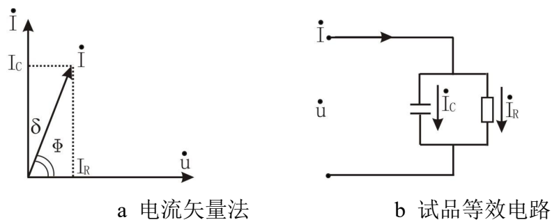
图 4 试品等效电路
