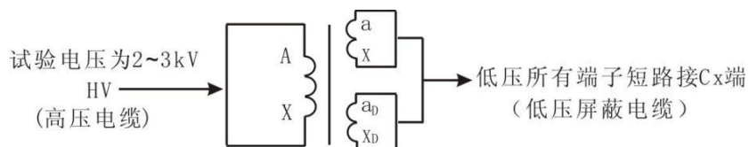
图 12 常规接线法
