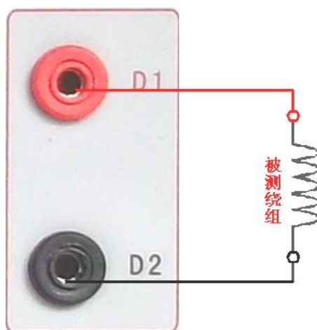
图 25，直阻测试接线图
