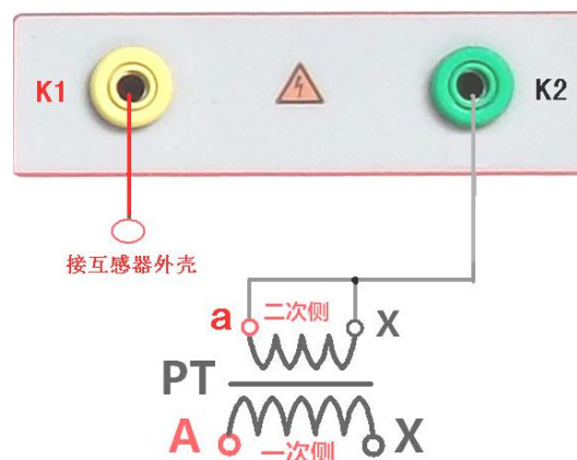
图 35, PT 交流耐压接线图
