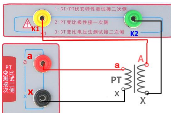
图 31, PT 变比极性（角差比差）接线图
