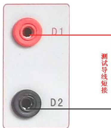
图 24，导线阻值清零接线图
