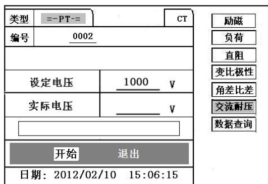
图 34, PT 交流耐压测试界面
