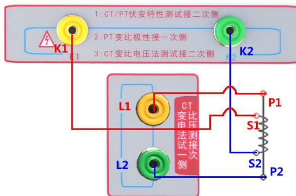
图 27 综合测试接线图
