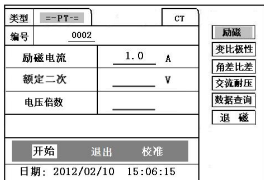
图 18, PT 励磁特性参数设置界面
