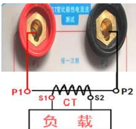
图 15、CT 一次通流接线图
