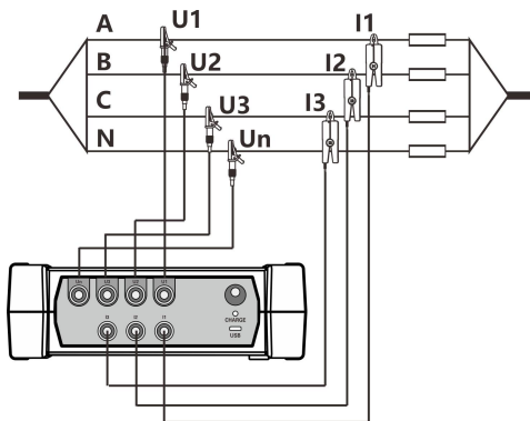
图 2（Y 型接线）
