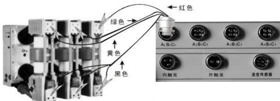
断口接线图（三断口）
