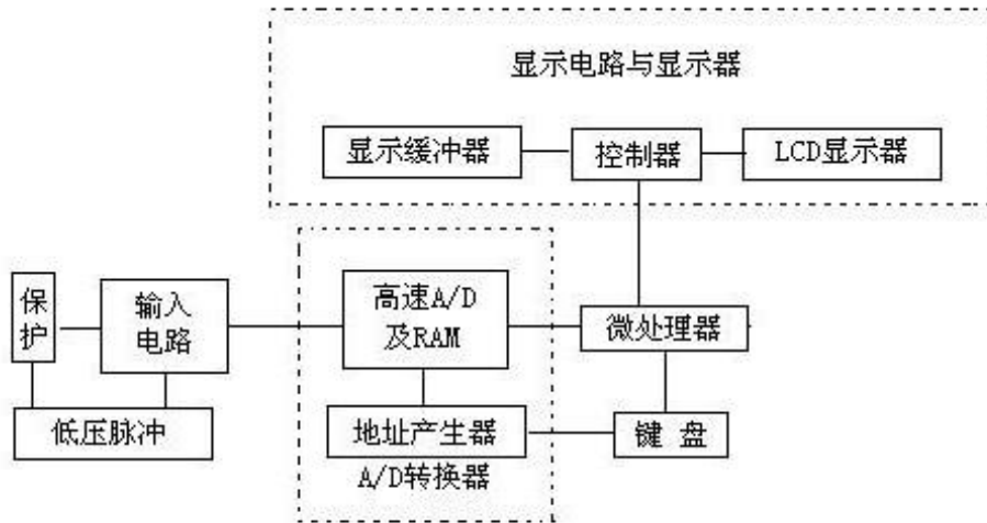
图 1 测试原理图
