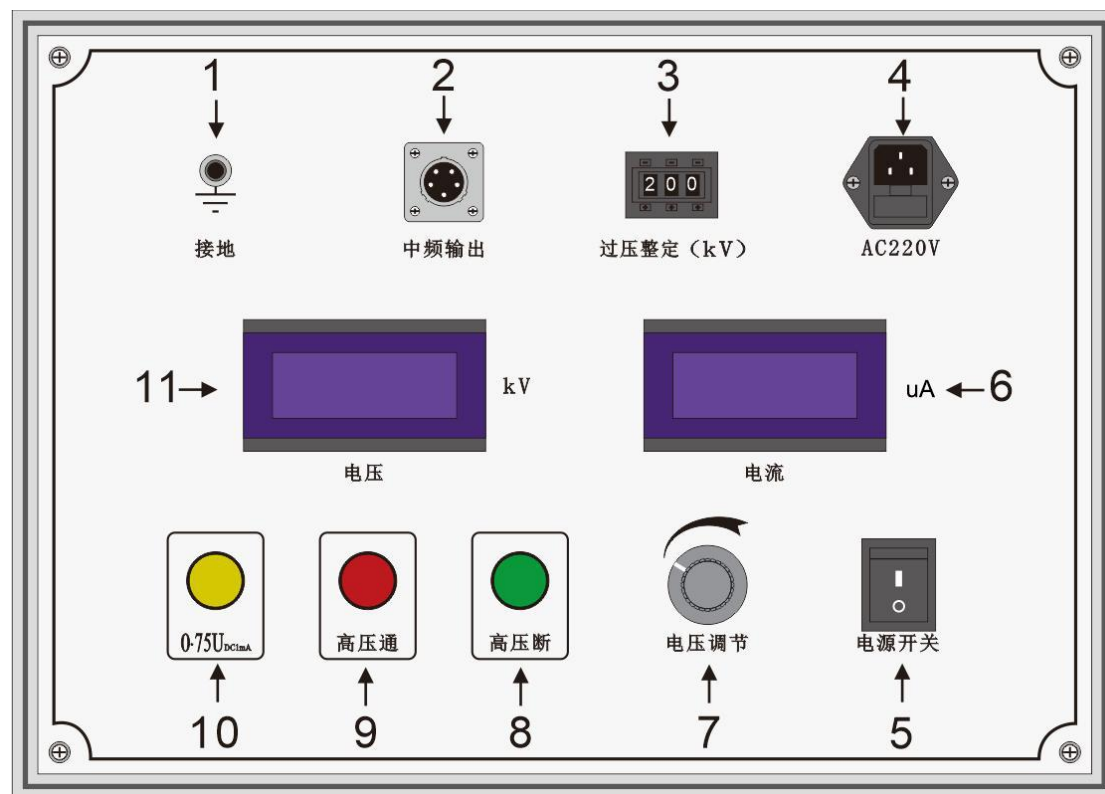
图 2 面板布局图
