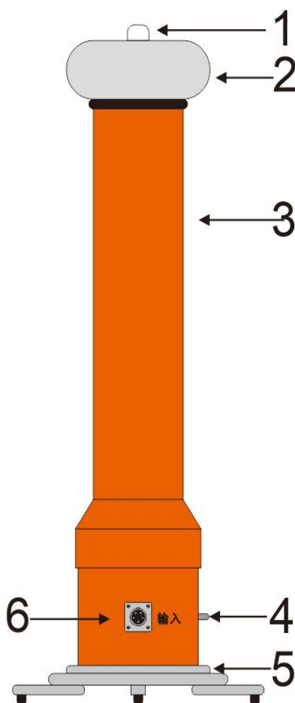
图 3 倍压筒示意图
