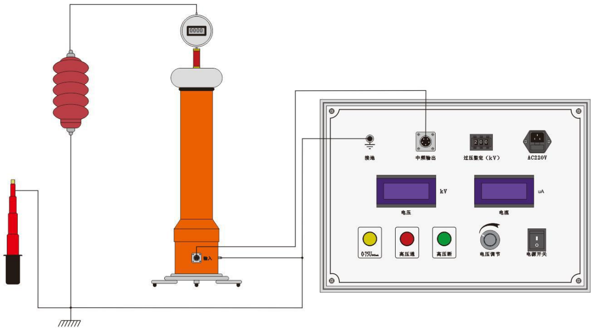
图 4 试验回路连接图
