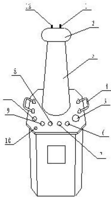
图 1：单台熔喷布静电驻极发生器外部结构图 图 2：单台熔喷布静电驻极发生器内部结构图
