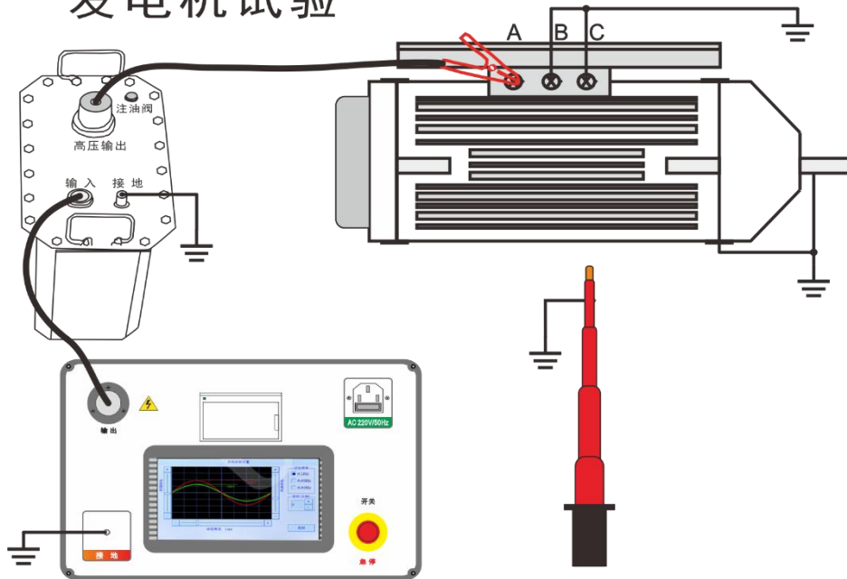
图 15 发电机试验接线示意图
