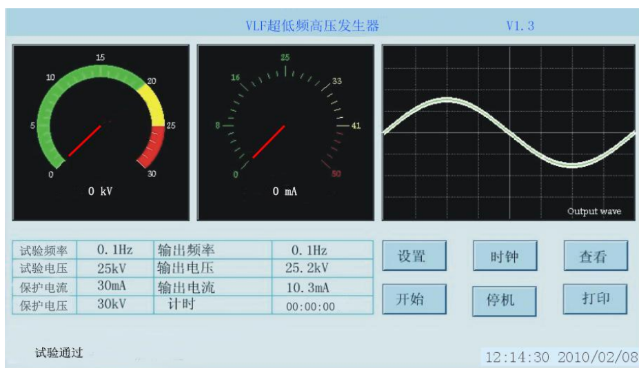
图 10 试验通过示意图
